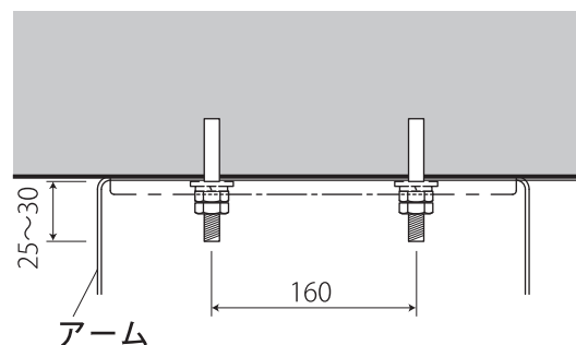
取付ボルト設置図
