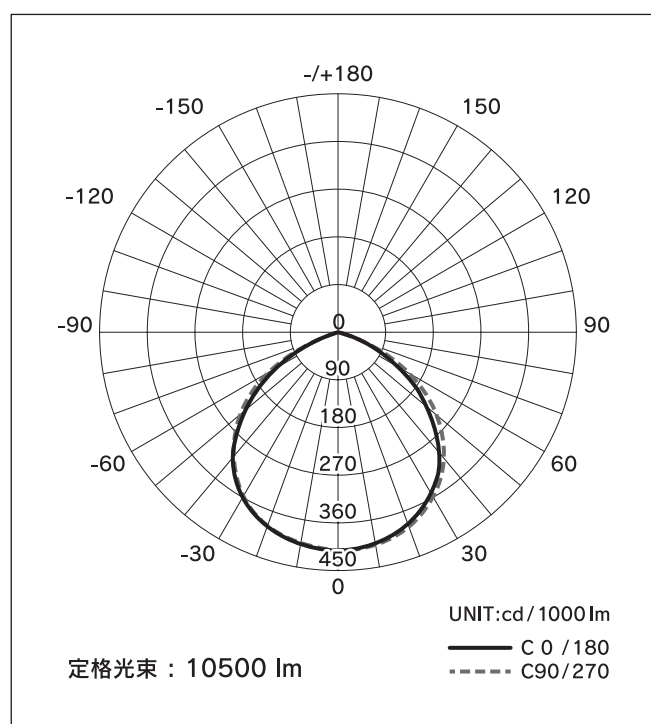
■配光曲線
