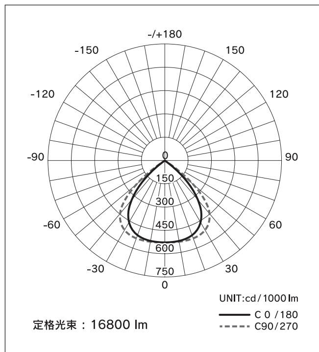
■配光曲線
