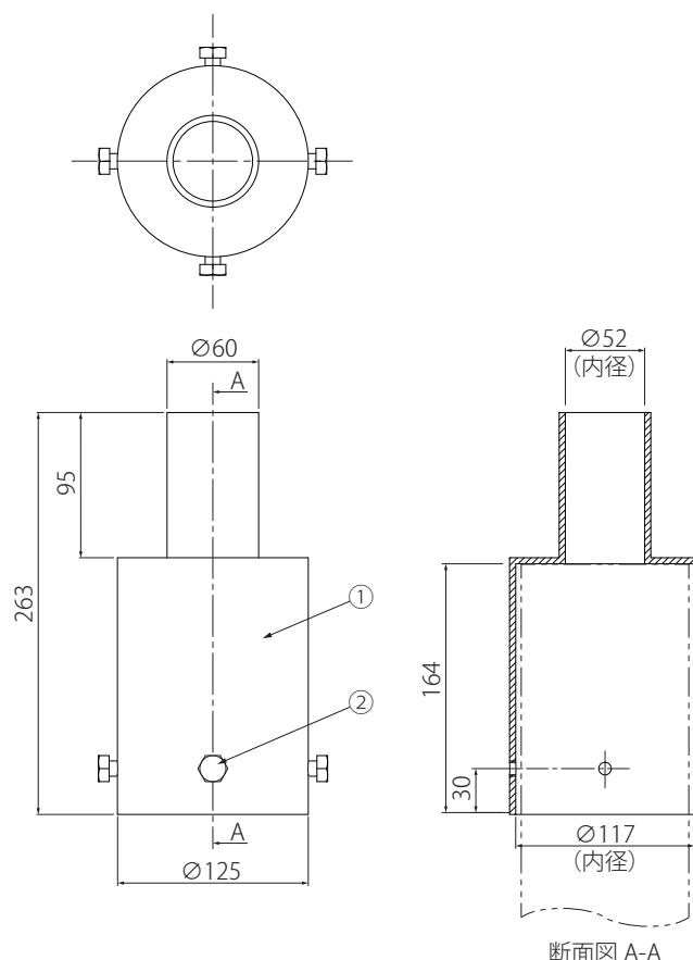
断面図 A-A
