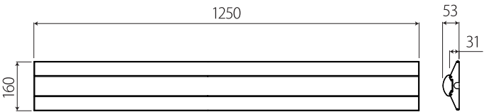
逆富士タイプ 幅160mm
